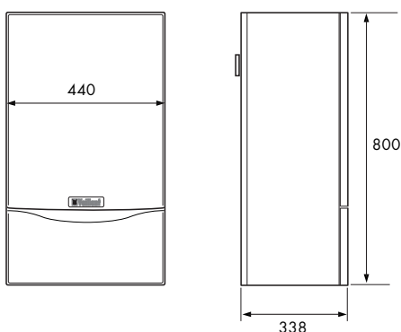
Габаритные размеры аппарата
