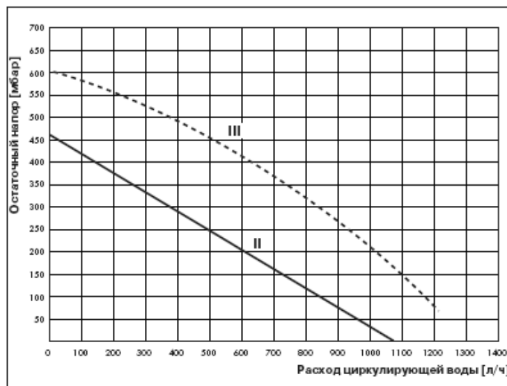
Характеристики насоса у аппарата Pro
