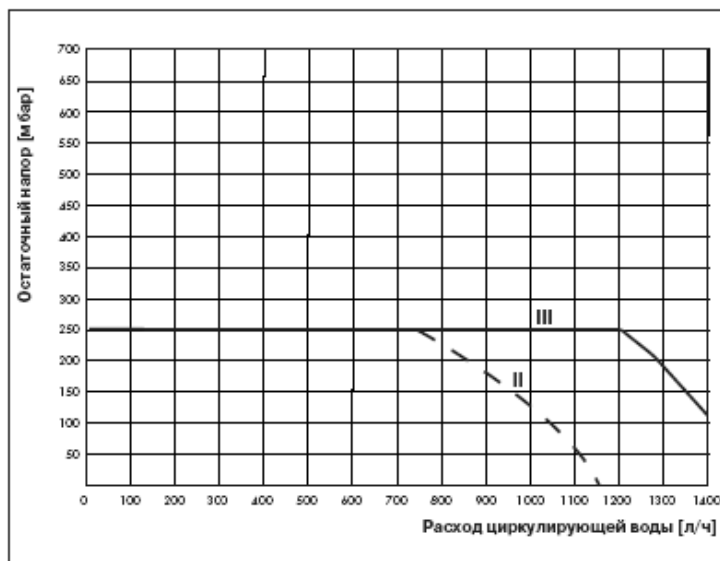
Характеристики насоса у аппарата Plus
