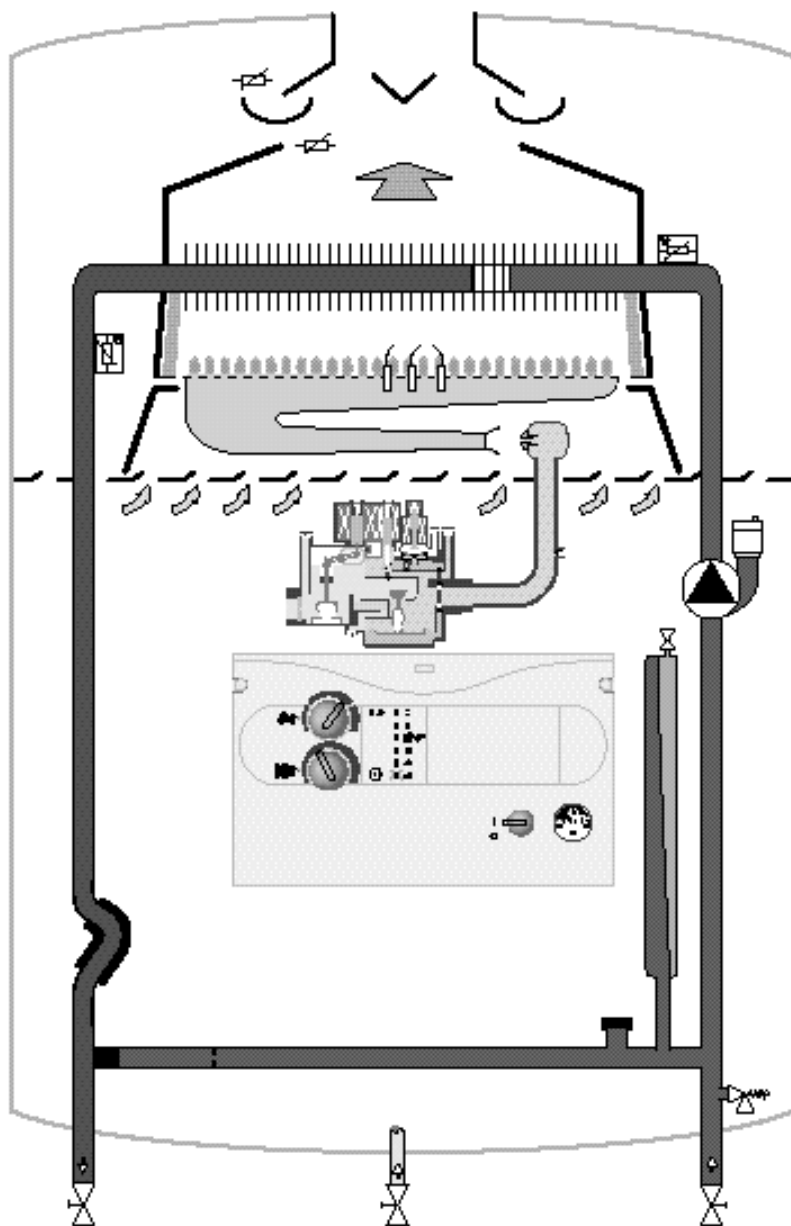
Функциональная схема atmoMAX Pro VU без встроенного приоритетного переключающего вентиля (Режим отопления)
