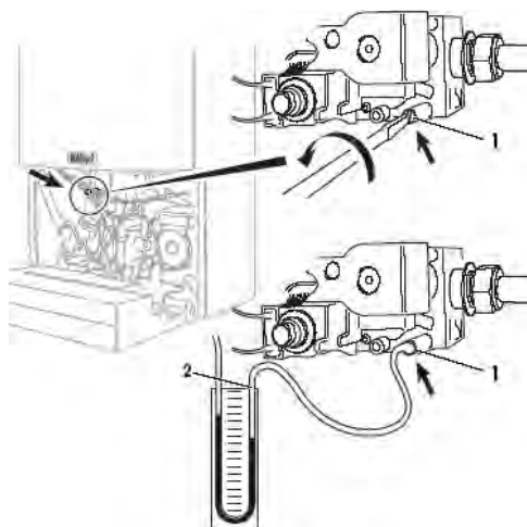
Проверка давления газа (давления истечения) в подводящем газопроводе
