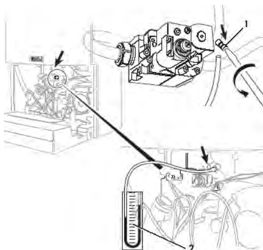
Присоединение U-образного манометра
