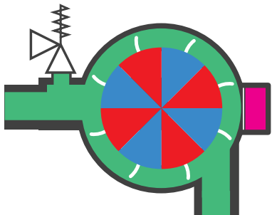
Датчик расхода воды (схема)
