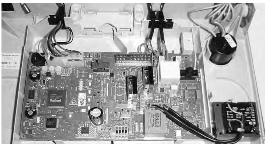
Электронный блок со снятыми крышками, вид сзади
