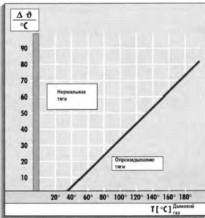
Характеристика дифференциального датчика отходящих газов
