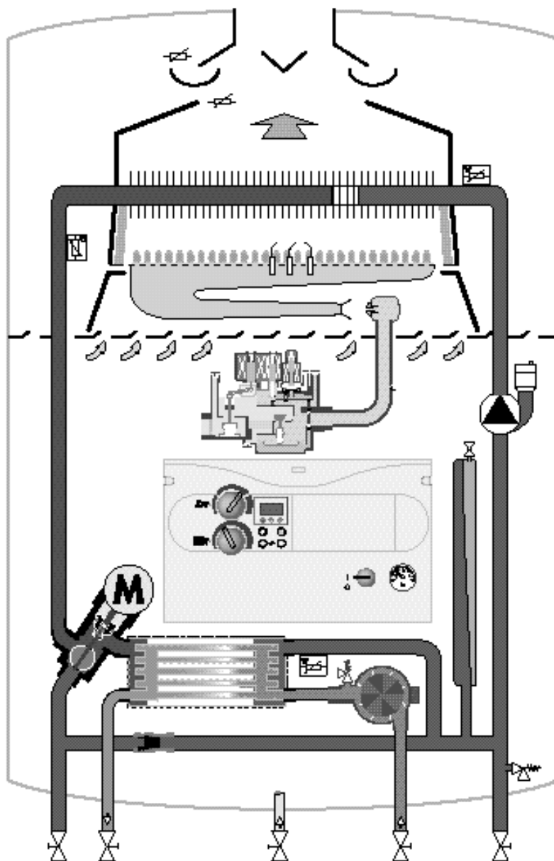
Функциональная схема atmoMAX Plus VUW (Режим отопления)
