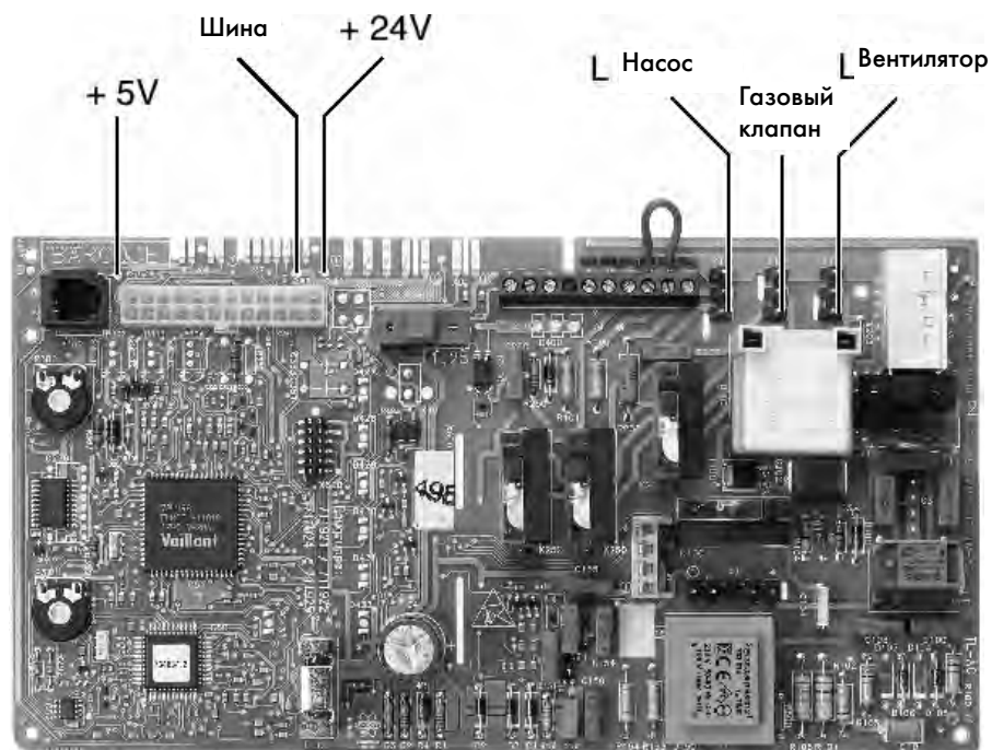
Контрольные точки на печатной плате
