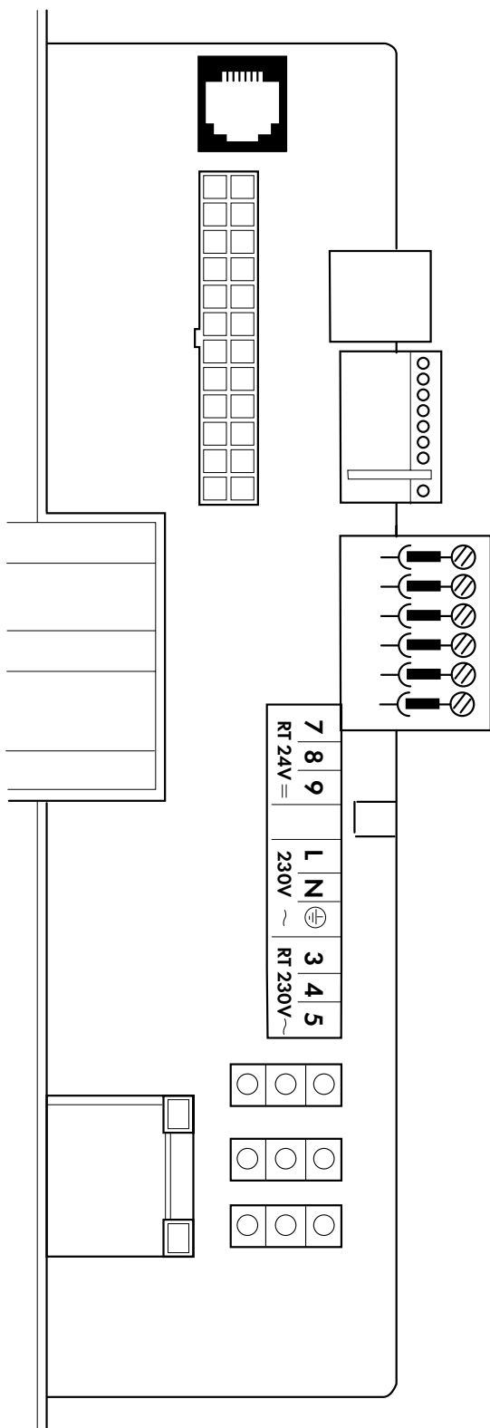
Клеммная колодка аппаратов.
